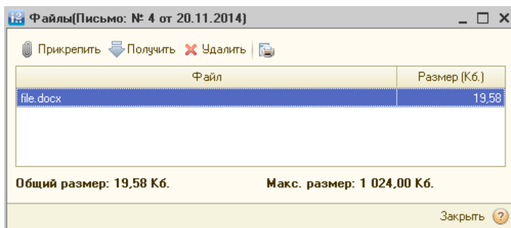
Рис. 53. Окно «Файлы»
